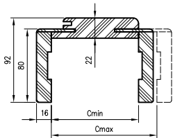
Przekrój OR z ką. T80
