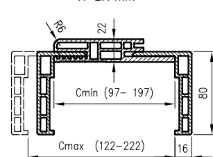
Przekrój belki ORB Water Proof dla Cmin 97-197 mm
