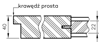
Przekrój poziomy drzwi Nestor
