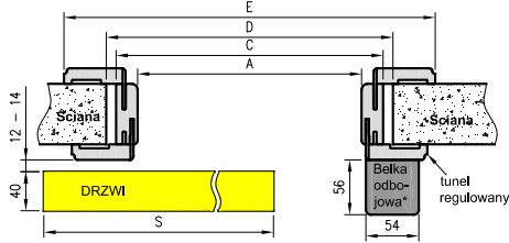
NT - przekrój poziomy (system lewy)
