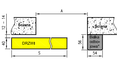
NS - przekrój poziomy (system lewy)
