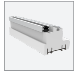
Ciepły próg aluminiowy z podwałiną podprogową klinarytową, h=35 mm
