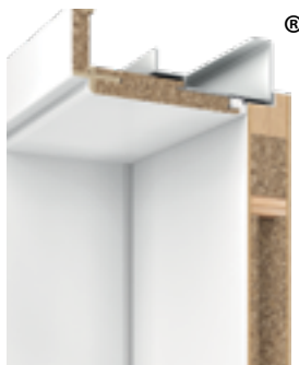
ościeżnica PROJEKT Premium
