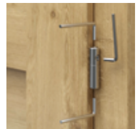
regulacja zawiasów czopowych regulowanych 3D
